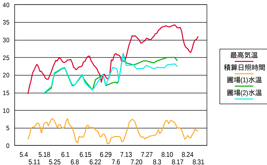
図１ アメダス築館の最高気温と水田水温（午前９時）の推移 １９９４年度 過去７日間の移動平均
