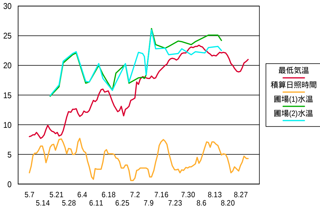
図2 アメダス築館の最低気温と水田水温(午前9時)の推移 1994年度 過去7日間の移動平均
