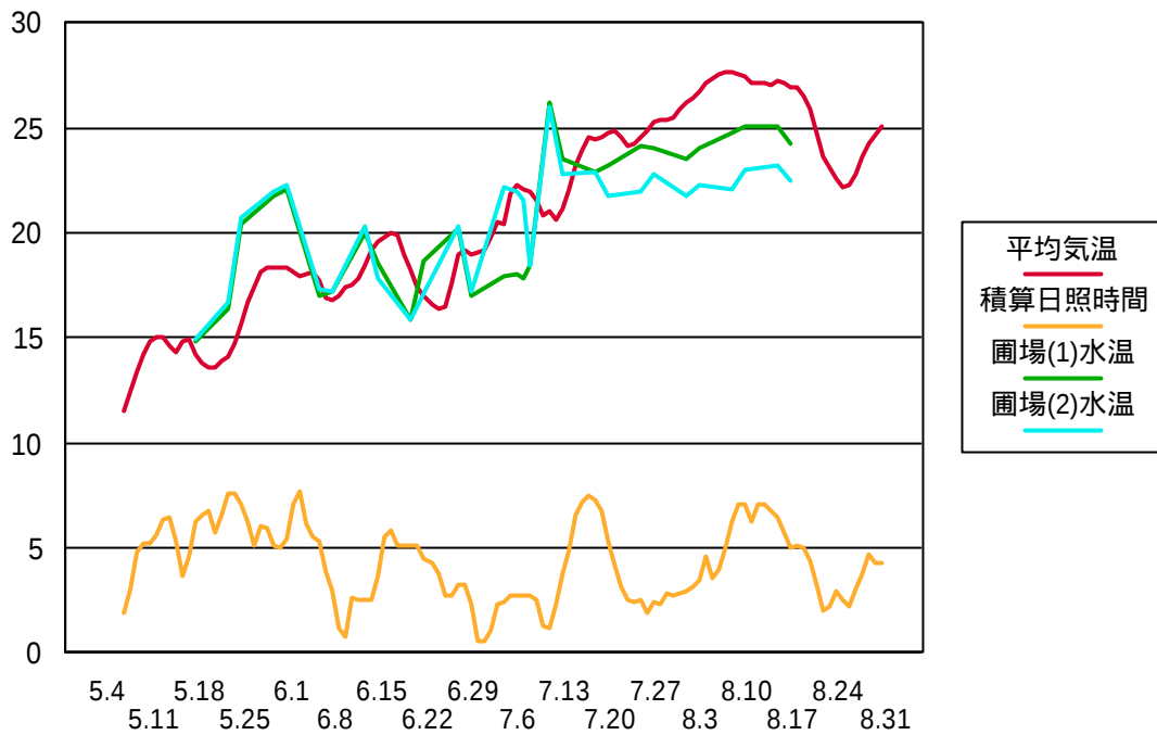
図3 アメダス築館の平均気温と水田水温 (午前9時)の推移 1994年度 過去7日間の移動平均
