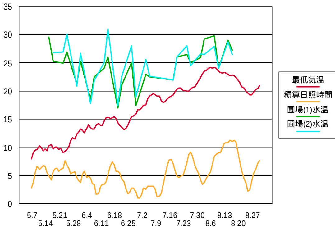
図2 アメダス浪江の最低気温と水田水温 (午前 9時)の推移 1994年度 過去 7日間の移動平均
