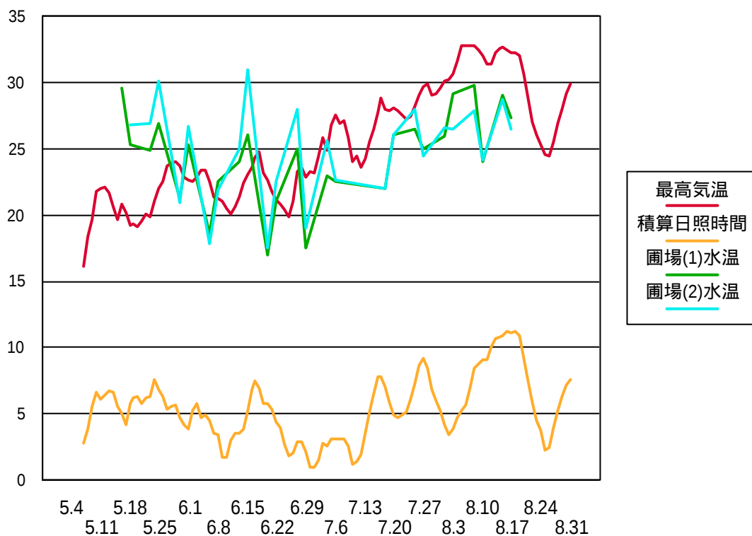
図１ アメダス浪江の最高気温と水田水温（午前９時）の推移 １９９４年度 過去７日間の移動平均
