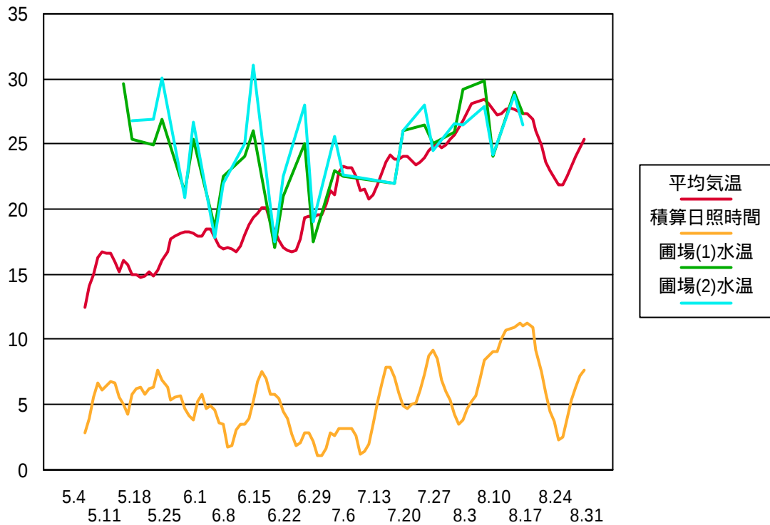
図3 アメダス浪江の平均気温と水田水温 (午前 9時 )の推移 1994年度 過去 7 日間の移動平均
