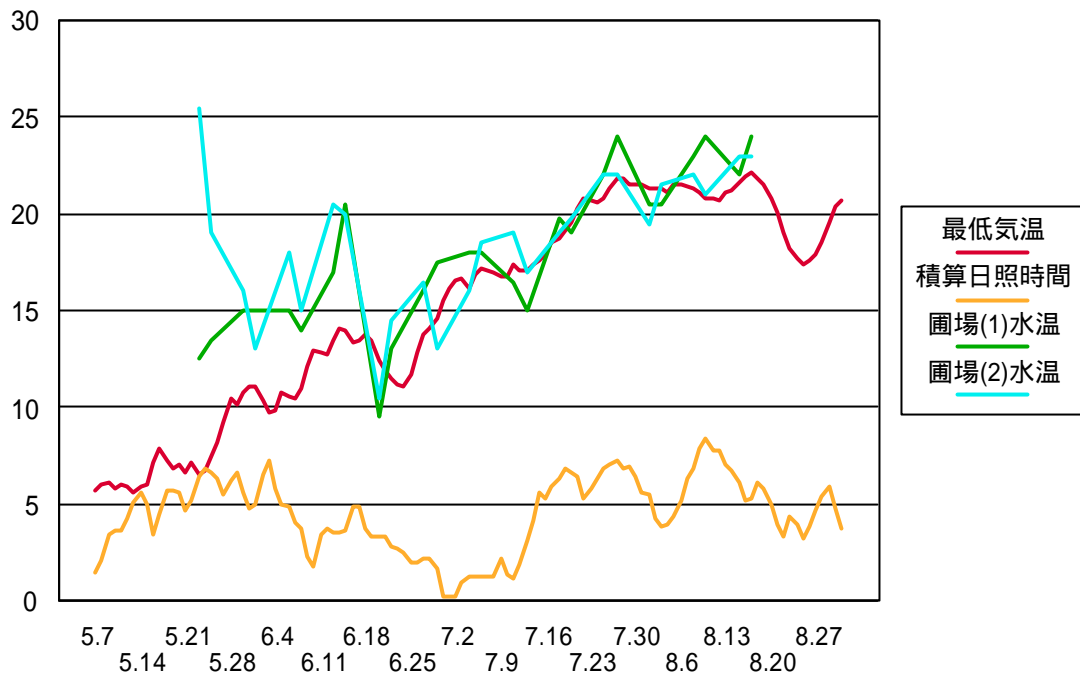
図2 アメダス遠野の最低気温と水田水温 (午前 9時 )の推移 1994年度 過去 7日間の移動平均
