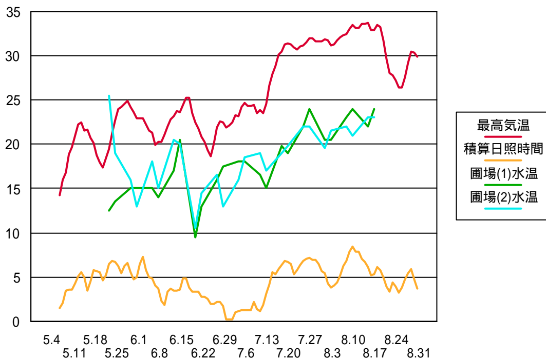
図１ アメダス遠野の最高気温と水田水温（午前９時）の推移 １９９４年度 過去７日間の移動平均
