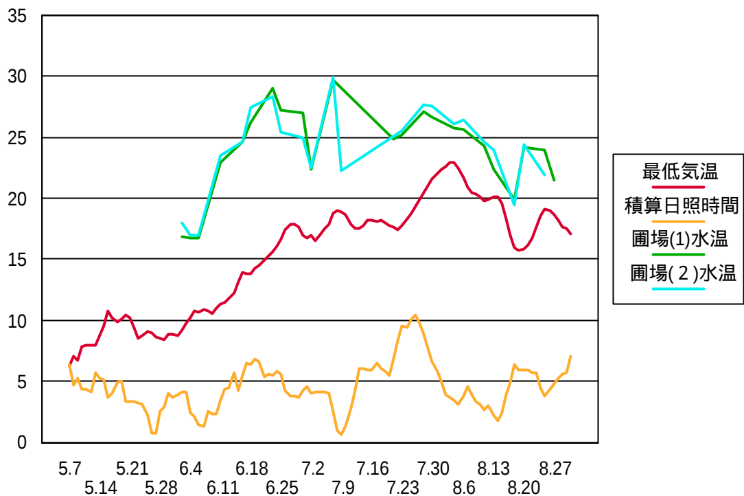
図2 アメダス弘前の最低気温と水田水温(午前9時)の推移 1997年度 過去7日間の移動平均
