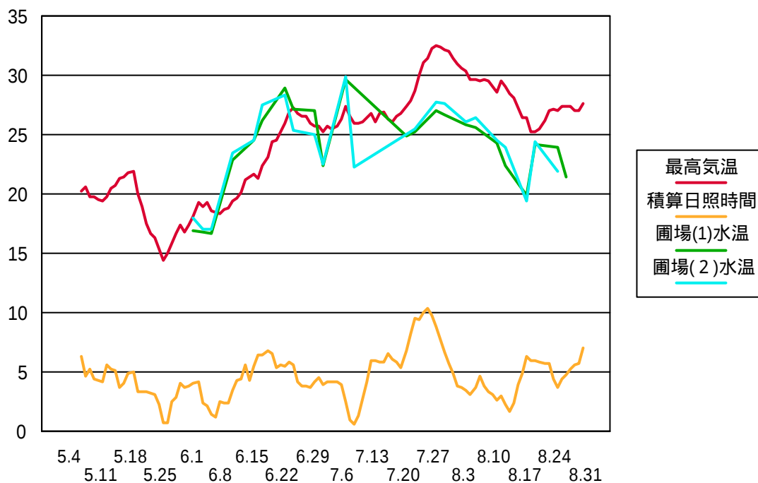
図１ アメダス弘前の最高気温と水田水温（午前９時）の推移 １９９７年度 過去７日間の移動平均
