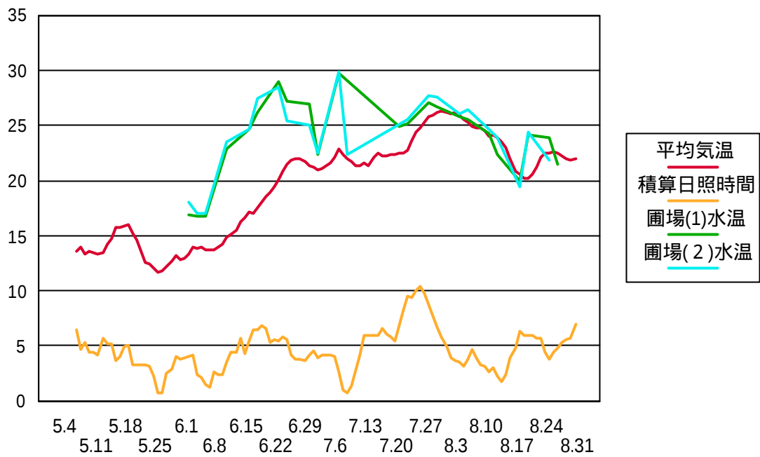
図3 アメダス弘前の平均気温と水田水温 (午前9時) の推移 1997年度 過去7日間の移動平均
